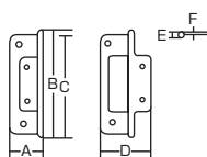
TS-113 クリーム ツキエス蝶番
